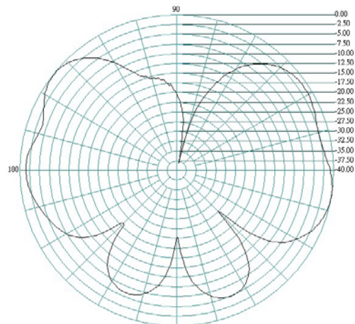
E-PLANE
